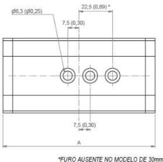
Figura 2.14 – Dimensional e montagem dos modelos de ímãs lineares.
